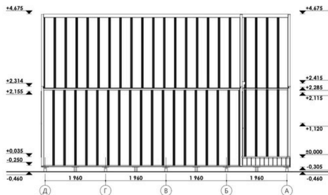
Façades
