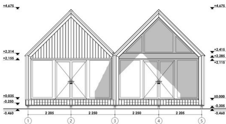
Façades
