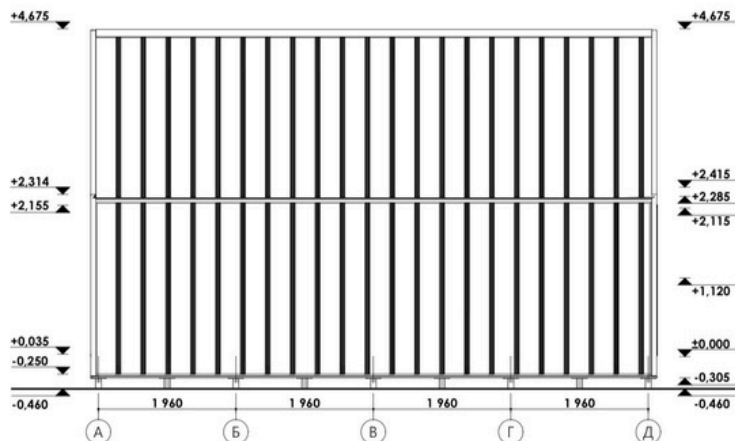
Façades
