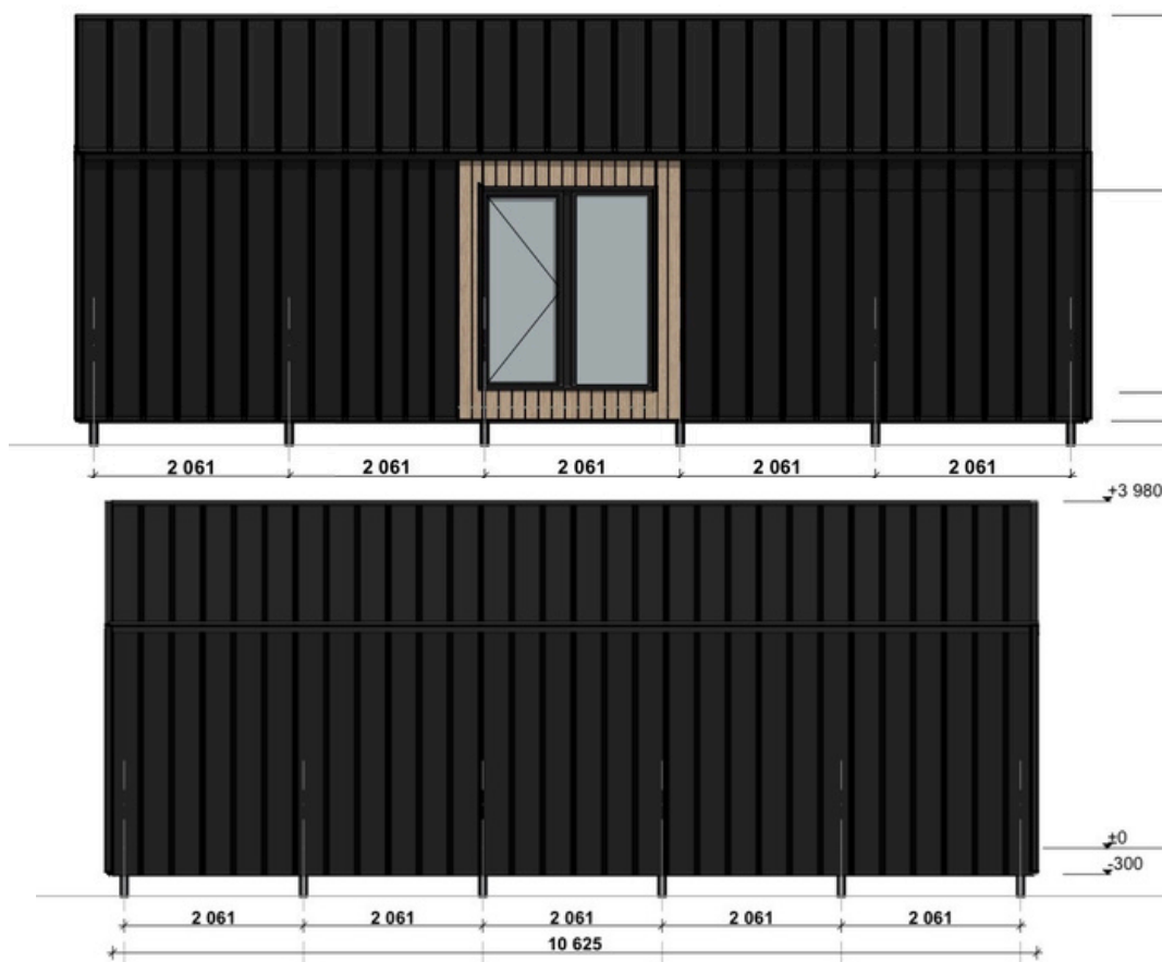
Façades Côtés
