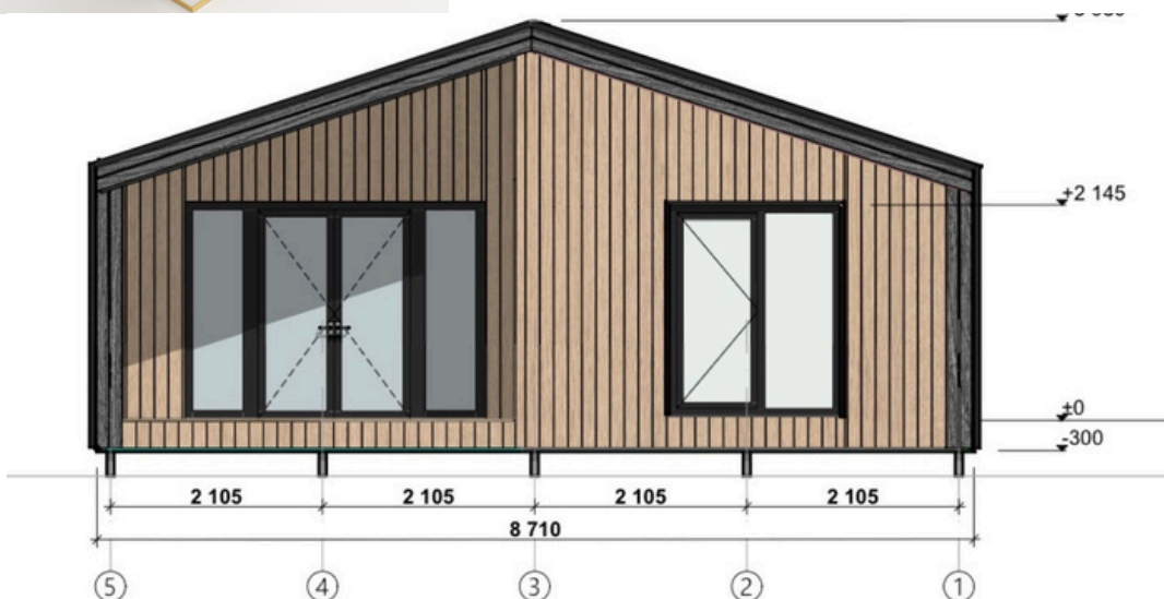
Façade Arrière
