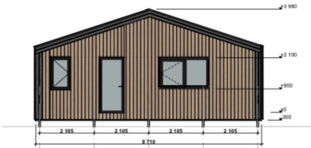
Façade Avant
