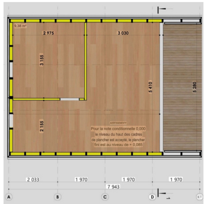
Maison à Ossature Bois : A-Frame
