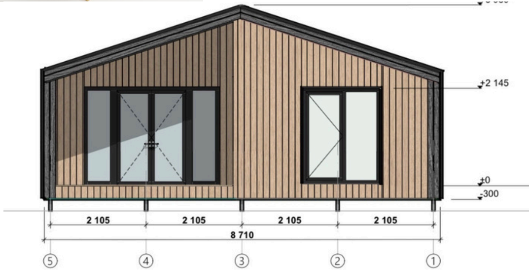
Façade Arrière
