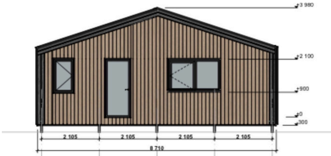
Façade Avant
