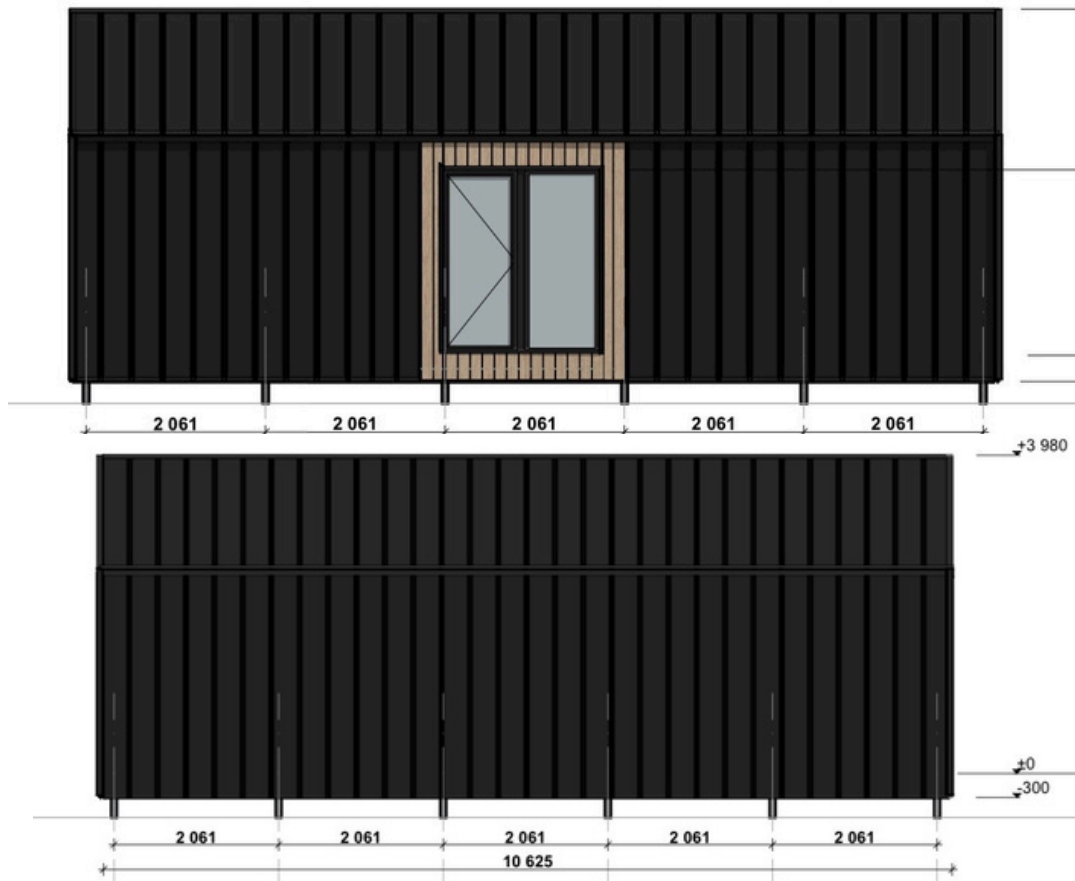
Façades Côtés
