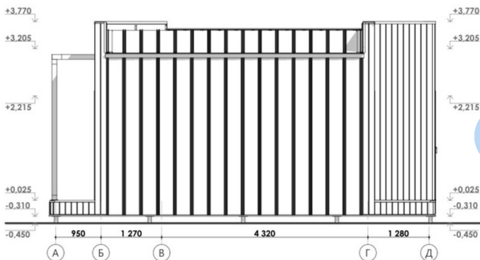
Façade Est
