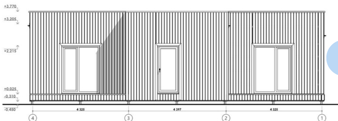
Façade Nord
