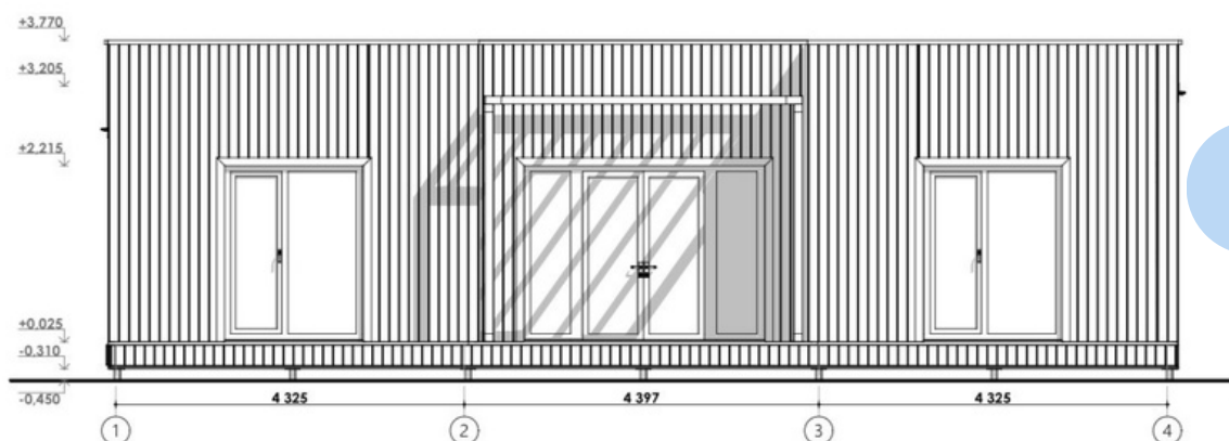
Façade Sud
